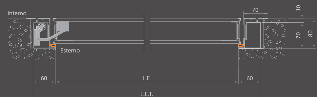
versione Complanare flush with wall
